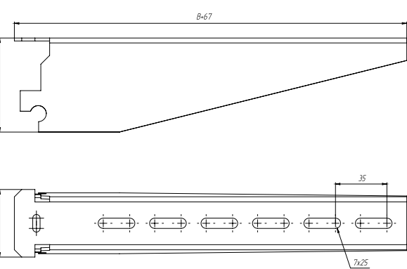
Полка кабельная
