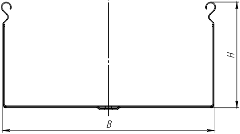
Габаритные размеры
