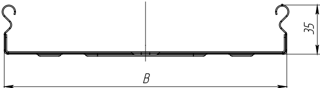
Габаритные размеры
