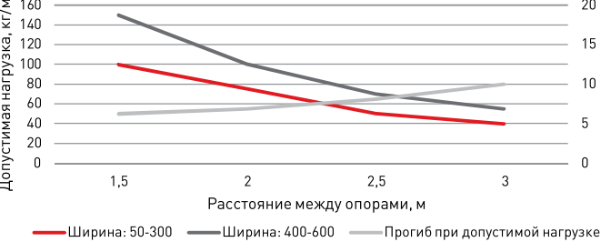
Графики нагрузки
