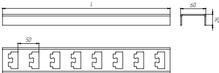
Стойка кабельная
