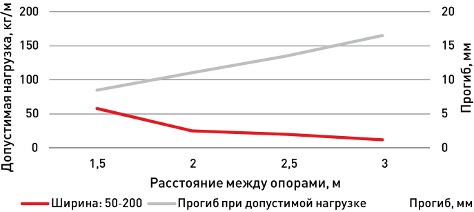
Графики нагрузки
