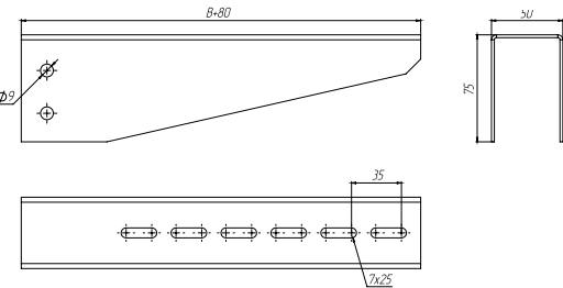
Кронштейн монтажный
