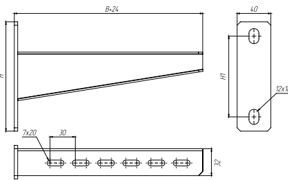
Консоль усиленная
