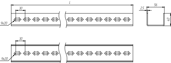
Профиль П-образный
