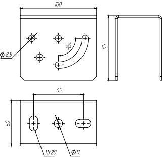
Скоба потолочная
