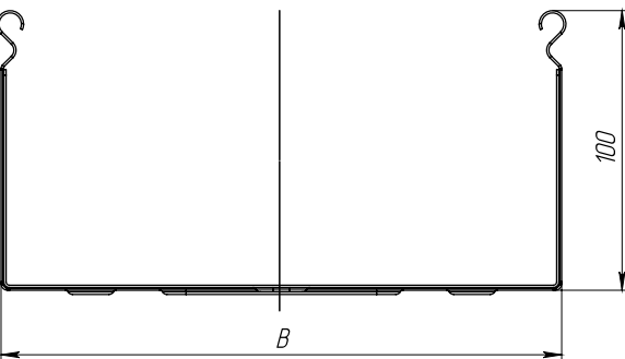
Габаритные размеры
