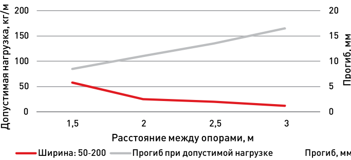
Графики нагрузки
