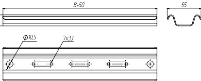
Омега-профиль
