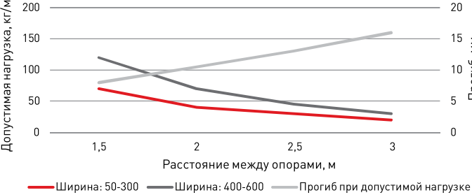
Графики нагрузки
