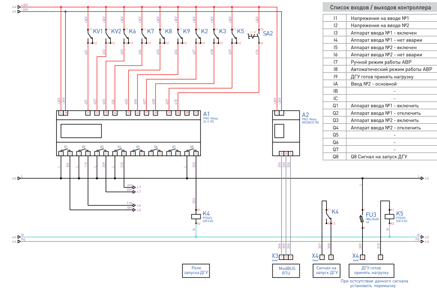
Схема электрическая подключения контроллера
