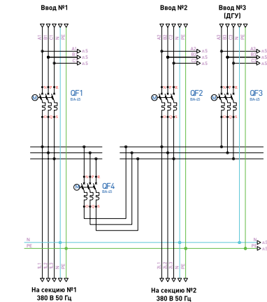
Пример электрической схемы АВР
