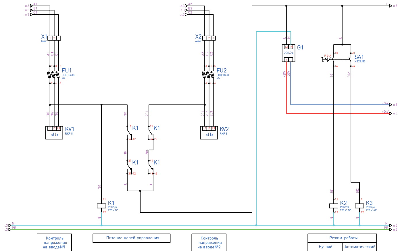
Схема электрическая подключения контроллера
